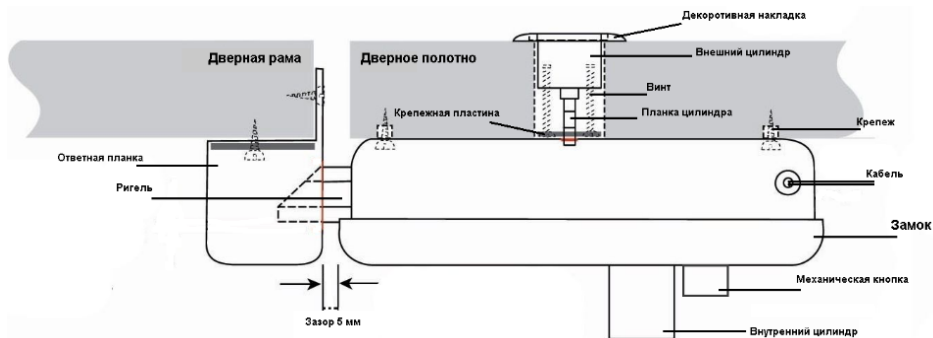
Рис. 9 Шаблон установки замка
