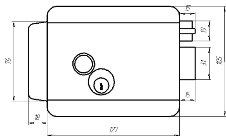
Рис. 1 Вид с лицевой стороны
