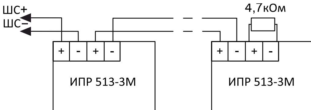
Рисунок 2.3. Схемы подключения извещателей в ШС прибора (продолжение)
