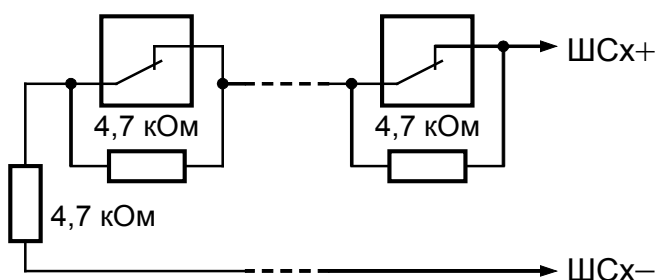
Рисунок 2.3. Схемы подключения извещателей в ШС прибора
