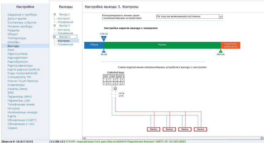
Рисунок 29. Контроль во включенном состоянии
