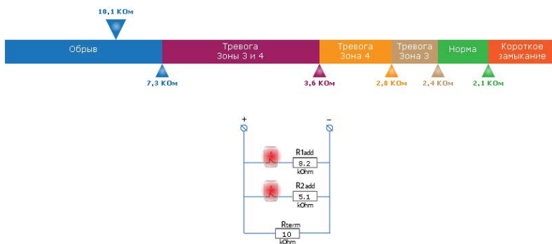
Рисунок 24. Шкала сопротивления резистивного шлейфа
