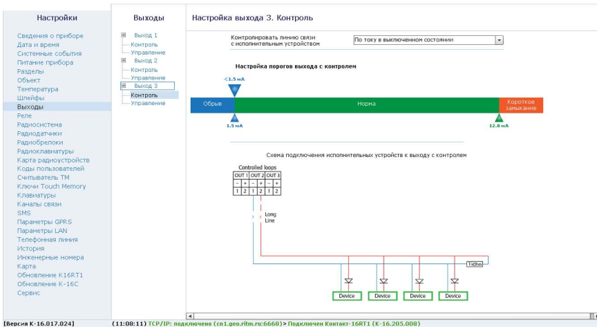
Рисунок 28. Контроль в выключенном состоянии
