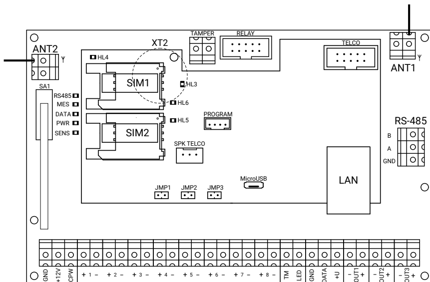
Рисунок 1. Лицевая сторона панели
