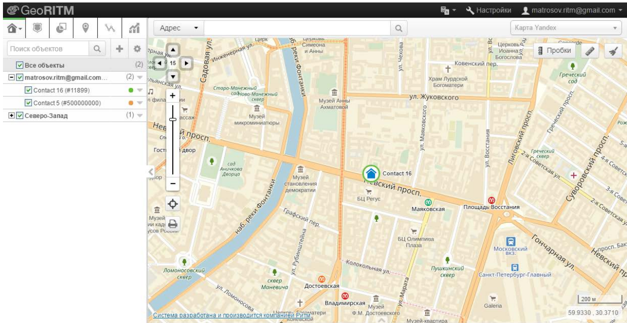
Рисунок 62. ПО GEO.RITM
