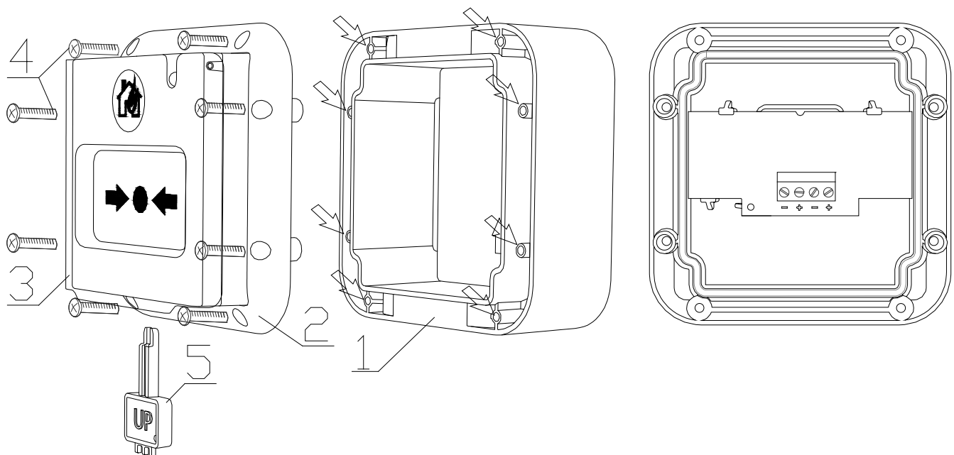
Рисунок 2.2.3.1 Основание ИПР
