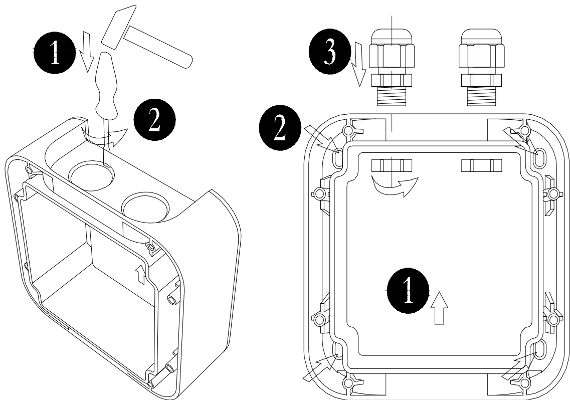
Рисунок 2.2.3.1 Основание ИПР
