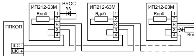
Рис.2 Типовая схема подключения извещателей для приборов с переполусовкой шлейфа сигнализации. Величина резисторов Rок и Rдоб определяется в соответствии с техническим описанием ППКОП.
