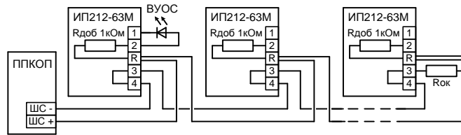
Рис.1 Типовая схема подключения извещателей для приборов с однополярным шлейфом сигнализации. Величина резистора Rок определяется в соответствии с техническим описанием ППКОП. Rдоб по умолчанию установлен – 1 кОм.
