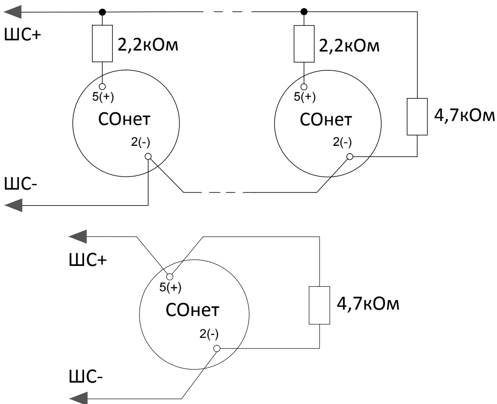
Схема подключения извещателей ИП435-8/101-04-А1R «СОНЕТ» в ШС типа 1 (сверху) и в ШС типа 2 (снизу)
