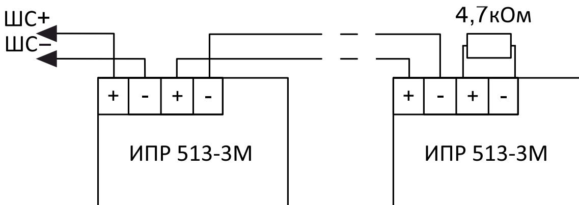
Схема подключения извещателей «ИПР 513-3М» ко входу дистанционного пуска
