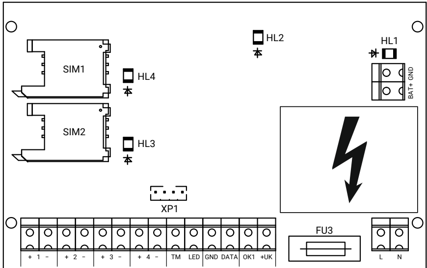
Рисунок 2. Контакт GSM-5A v.1
